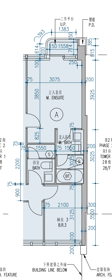
28/F Unit A Part Plan 28樓A單位之部分平面圖
