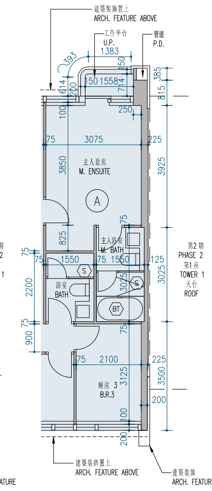
29/F Unit A Part Plan 29樓A單位之部分平面圖
