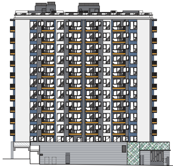
Elevation 2 立面圖2
