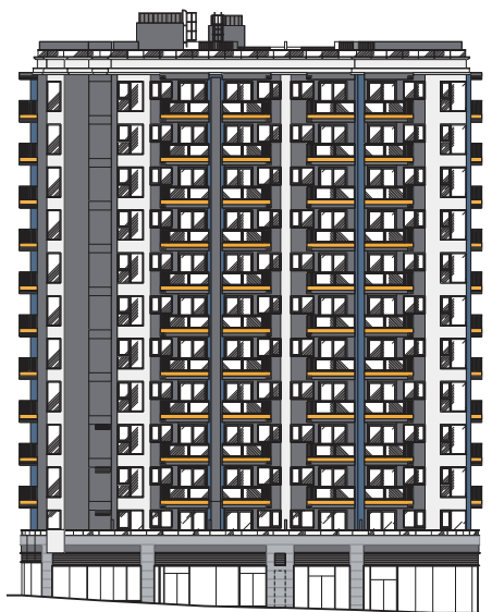
Elevation 2 立面圖2
