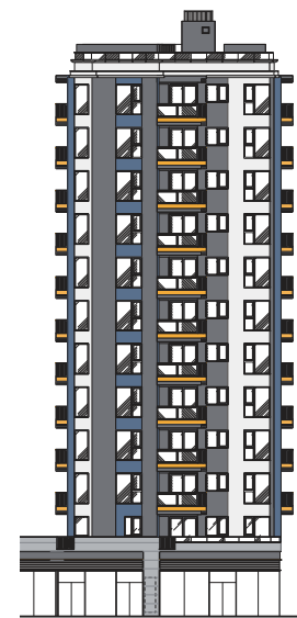
Elevation 4 立面圖4
